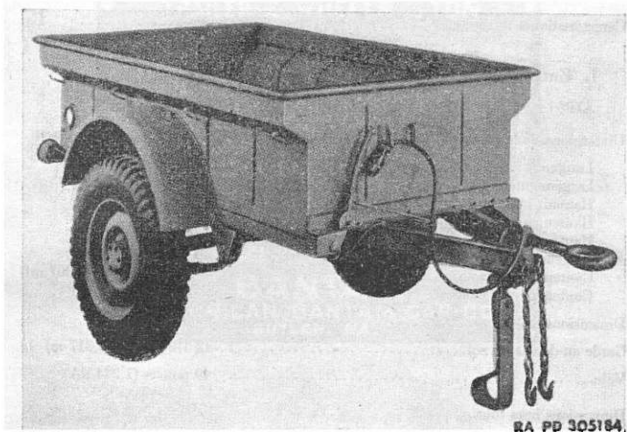
FIGURE 1. — Remorque de 1/4 tonne.
