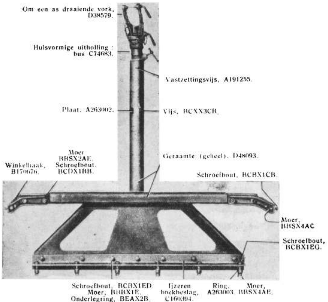
Fig. 1. — Affuitvoetstuk M24A1 voor vrachtwagens.
